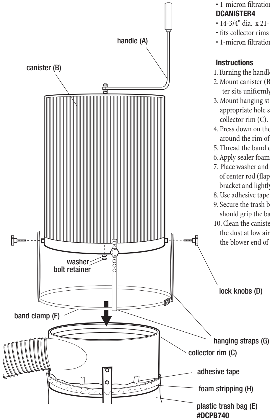
Fig. A- Assembly
